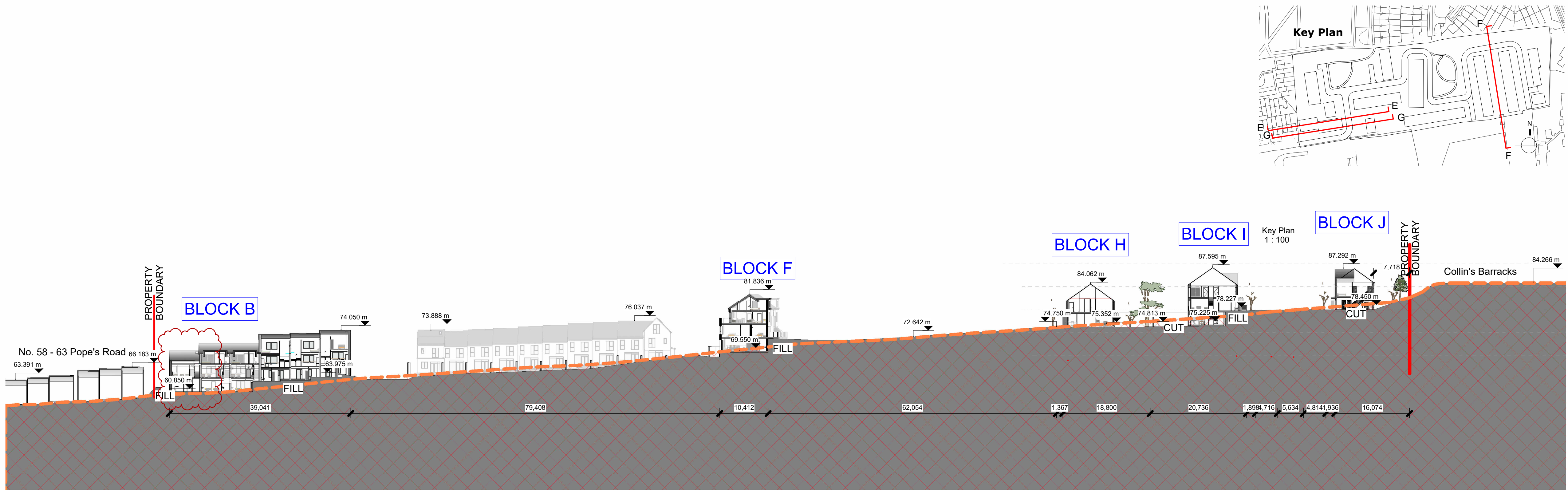
Section E-E 1 : 500
