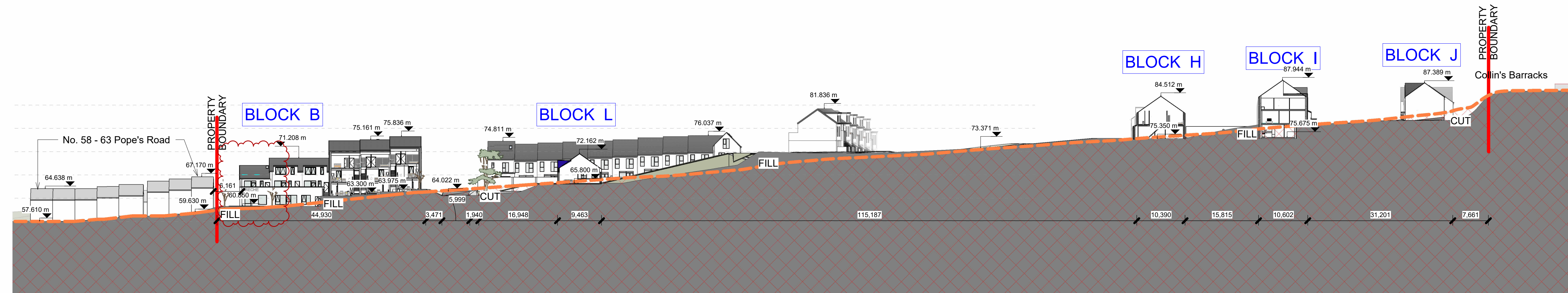
Section G-G 1 : 500
